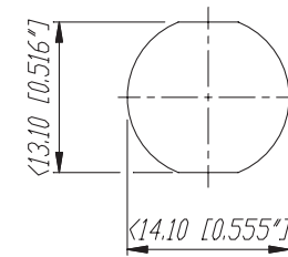
Frontplattenausschnitt (Rückseite) Panel cut out (rear side)
