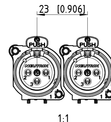
min. Einbauabstand min assembling distance
