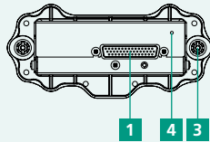
MODULE / top view
